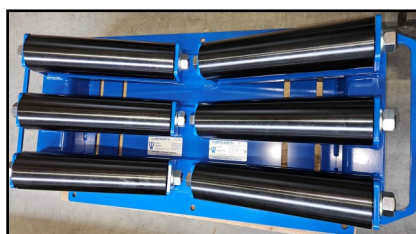
Uitvoering met totaal 6 rollen voor in LENGTE rollen van pijp. Extra draagvermogen door de 2 x 3 rollen. Model WRB-E-4-48-HD
